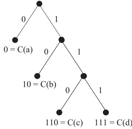
Figura 2.1: Árvore binária associada ao código instantâneo definido por C(a) = 0 , C(b) = 10 , C(c) = 110 , C(d) = 111 .
