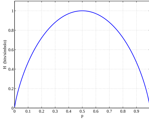
Figura 1.1: Entropia de uma fonte binária sem memória em função da probabilidade de um dos símbolos.
